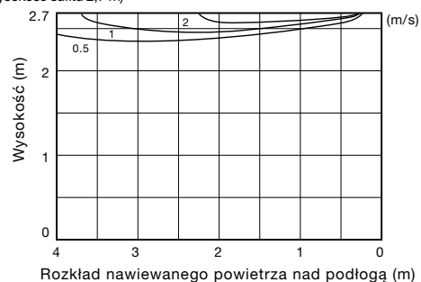
SLZ-M60FA Nawiew powietrza pod kątem, praca w trybie chłodzenia przy 20°C (wysokość sufitu 2,7 m)
